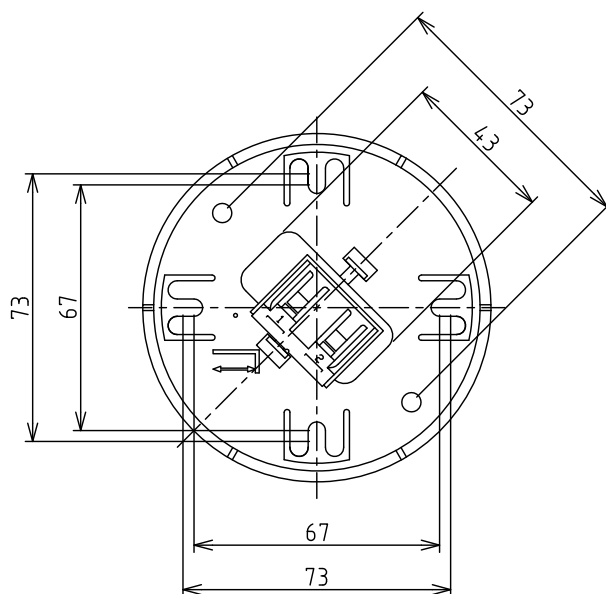
取付寸法図
