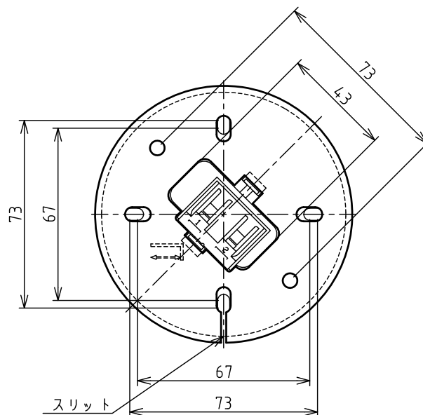
取付寸法図
