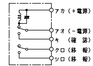
内部回路図 (作動前)
