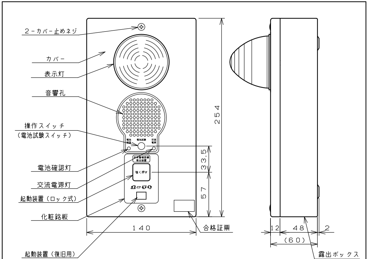
通線孔及び取付孔位置 (正面図)
