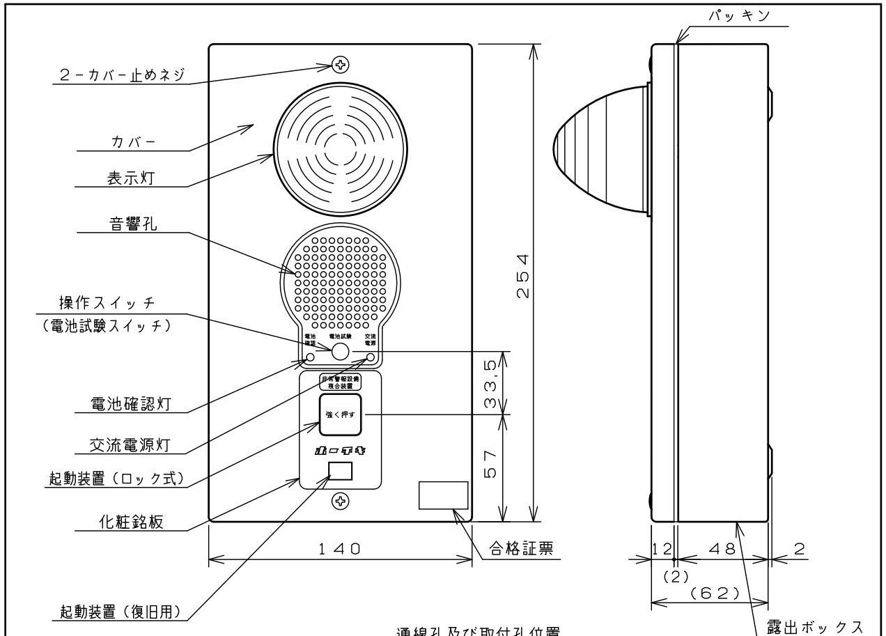
通線孔及び取付孔位置 (正面図)
