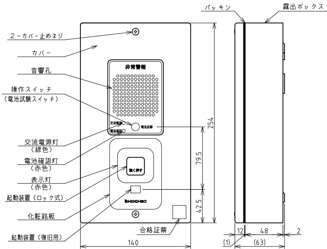
通線孔および取付孔位置 (正面図)
