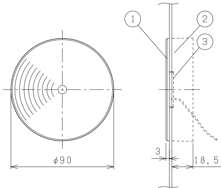
板金取付図 (フラット取付)
