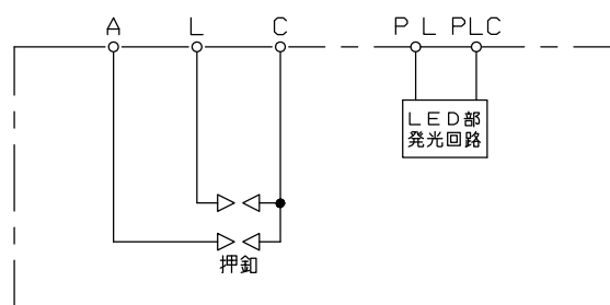
回路図
