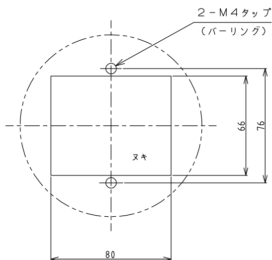
取付寸法図
