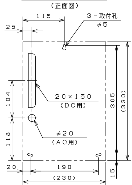
通線孔位置及び取付孔位置
