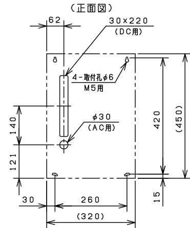
通線孔位置及び取付孔位置
