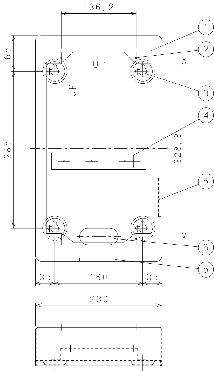
取付穴寸法図 S=1/2
