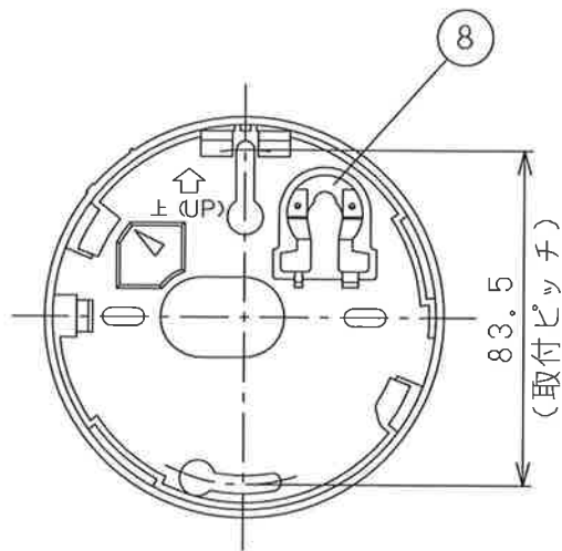
取付寸法図
