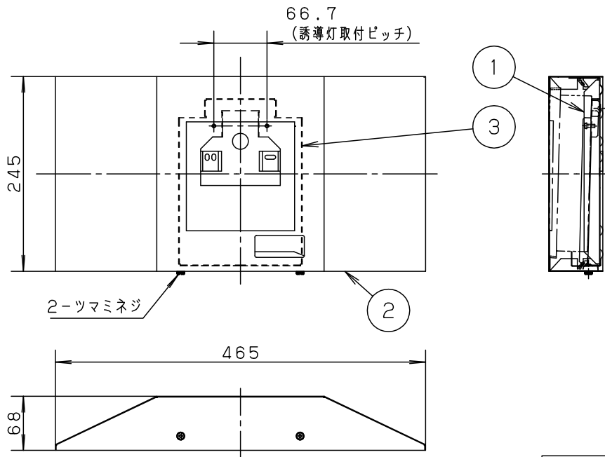
背面図
