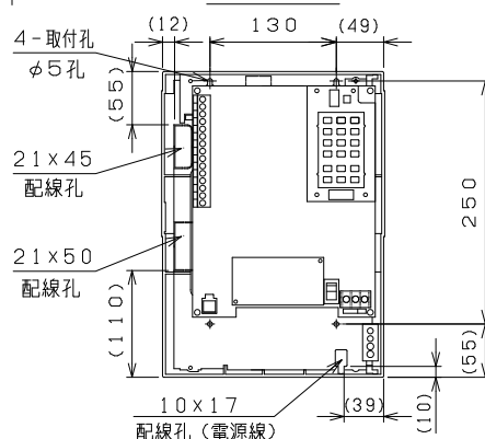
取付寸法図
