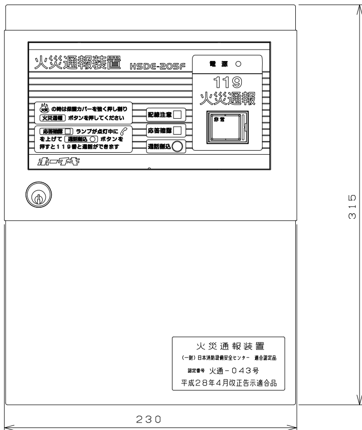
取付寸法図
